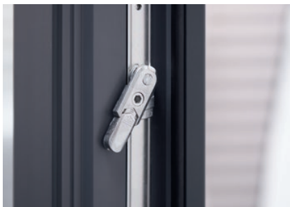
Zasuwnica z blokadą obrotu klamki i podnośnikiem skrzydła
