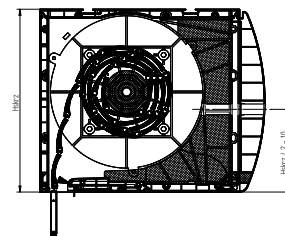
■ Skrzynka prosta z nawiewnikiem
