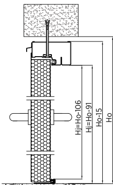
Rys. 124. Montaż do muru drzwi jednoskrzydłowych - ościeżnica wewnętrzna z przekładką termiczną - przekrój pionowy
