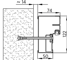
Rys. 68. Ościeżnica wewnętrzna z przekładką termiczną
