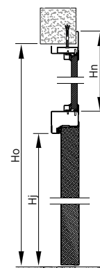
Rys. 105. Naświetle górne - przekrój pionowy
