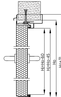
Rys. 120. Montaż do muru drzwi jednoskrzydłowych – ościeżnica obejmująca z przekładką termiczną – przekrój pionowy
