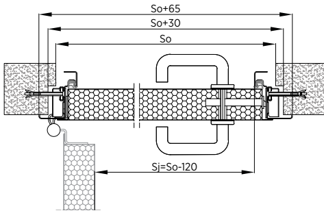
Rys. 115. Montaż do muru drzwi jednoskrzydłowych – ościeżnica narożna z przekładką termiczną – przekrój poziomy
