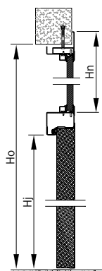
Rys. 102. Naświetle górne - przekrój pionowy
