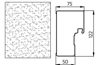
Rys. 29. Ościeżnica wewnętrzna
