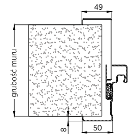
Rys. 33. Ościeżnica obejmująca z przekładką termiczną
