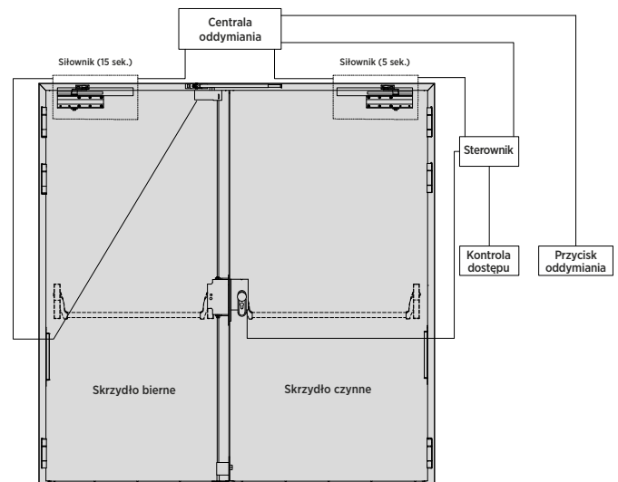
Rys. 100. Schemat podłączenia elementów układu napowietrzania drzwi stalowych płaszczykowych dwuskrzydłowych z funkcją paniczną
