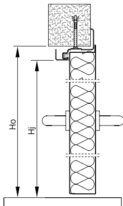
Rys. 175. Montaż na ścieżnicy narożnej – przekrój pionowy.
