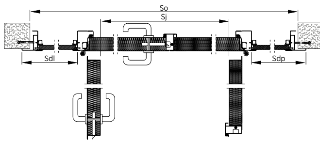
Rys. 106. Doświetla boczne - przekrój poziomy
