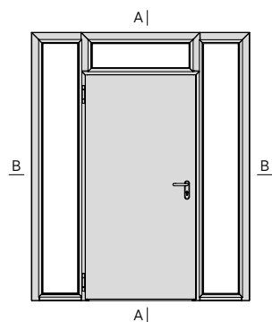
Rys. 101. Drzwi jednoskrzydłowe ECO z doświetlami bocznymi i naświetlem górnym
