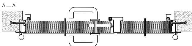
Rys. 64. Przekrój poziomy na wysokości zamka drzwi stalowych płaszczyznych zewnętrznych ECO z ościeżnicą narożną bez przekładki termicznej
