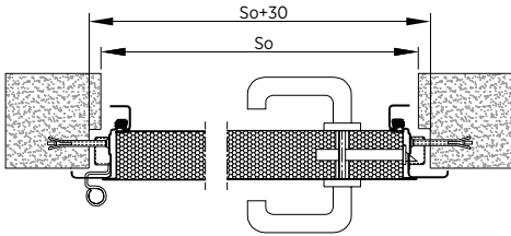
Rys. 107. Montaż do muru drzwi jednoskrzydłowych z ościeżnicą narożną bez przekładki termicznej - przekrój poziomy
