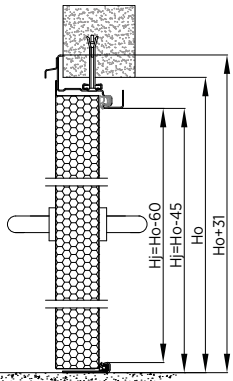
Rys. 116. Montaż do muru drzwi jednoskrzydłowych – ościeżnica narożna z przekładką termiczną – przekrój pionowy
