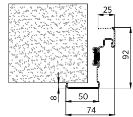
Rys. 31. Ościeżnica narożna z przekładką termiczną
