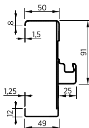
Rys. 159. Ościeżnica obejmująca
