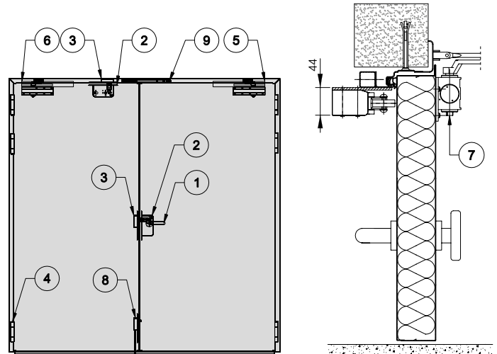
Rys. 98. Schemat drzwi dwuskrzydłowych – przekrój pionowy z układem napowietrzania
