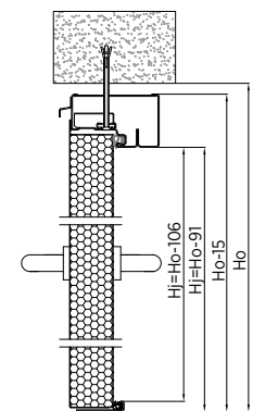
Rys. 126. Montaż do muru drzwi dwuskrzydłowych - ościeżnica wewnętrzna z przekładką termiczną - przekrój pionowy
