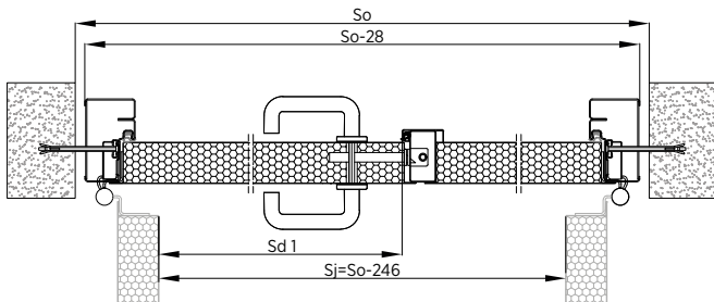
Rys. 125. Montaż do muru drzwi dwuskrzydłowych - ościeżnica wewnętrzna z przekładką termiczną - przekrój poziomy
