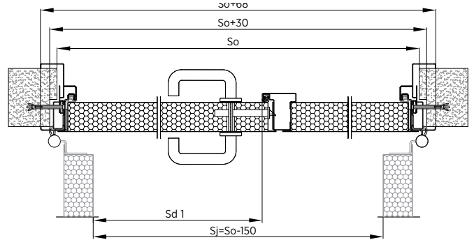
Rys. 121. Montaż do muru drzwi dwuskrzydłowych – ościeżnica obejmująca z przekładką termiczną – przekrój poziomy
