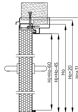
Rys. 122. Montaż do muru drzwi dwuskrzydłowych – ościeżnica obejmująca z przekładką termiczną – przekrój pionowy
