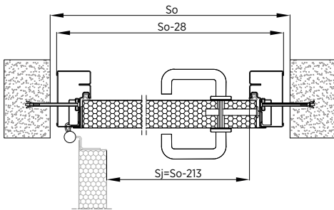
Rys. 123. Montaż do muru drzwi jednoskrzydłowych - ościeżnica wewnętrzna z przekładką termiczną - przekrój poziomy
