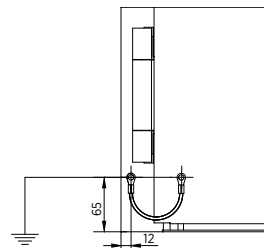
Rys. 96. Sposób wykonania uziemienia drzwi ECO
