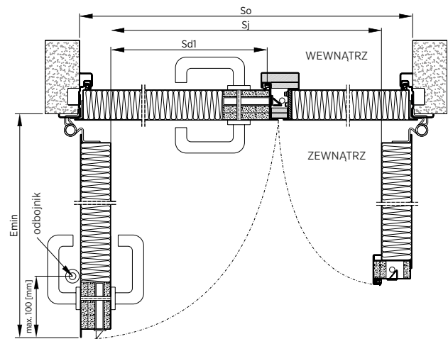
Rys. 177. Montaż na ścieżnicy narożnej drzwi dwuskrzydłowych – przekrój poziomy
