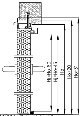
Rys. 118. Montaż do muru drzwi dwuskrzydłowych – ościeżnica narożna z przekładką termiczną – przekrój pionowy
