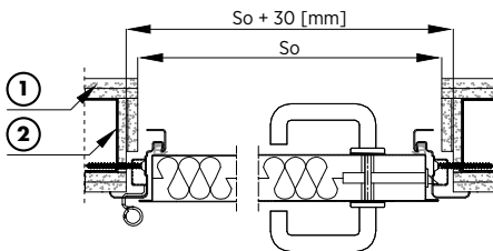
Rys. 169. Montaż do muru drzwi jednoskrzydłowych z ościeżnicą narożną – przekrój poziomy
