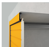
Montaggio nel foro - carter nel foro
