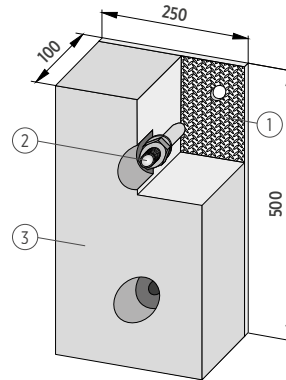
Butoir avec platine.
