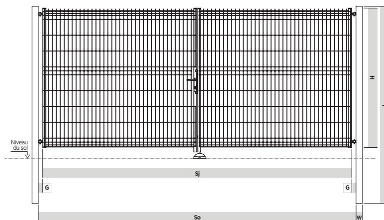
Portail à deux battants MODEST vue de l'intérieur
