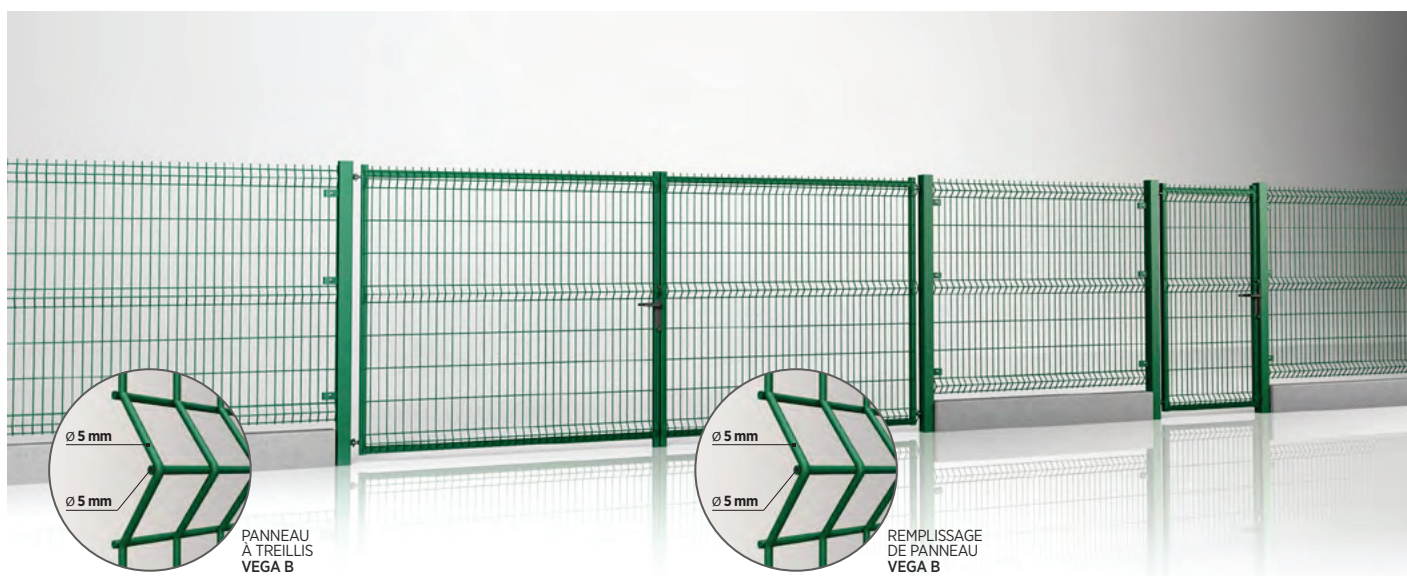
Clôture systémique avec portail à deux battants et portillon MODEST - remplissage d'un panneaux à treillis Vega B
