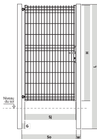
Portillon MODEST vue de l'intérieur
