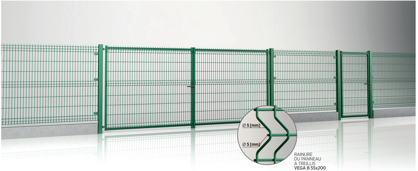
Clôture systémique avec portail et portillon MODEST avec remplissage en panneaux à treillis VEGA B, maille 55x200
