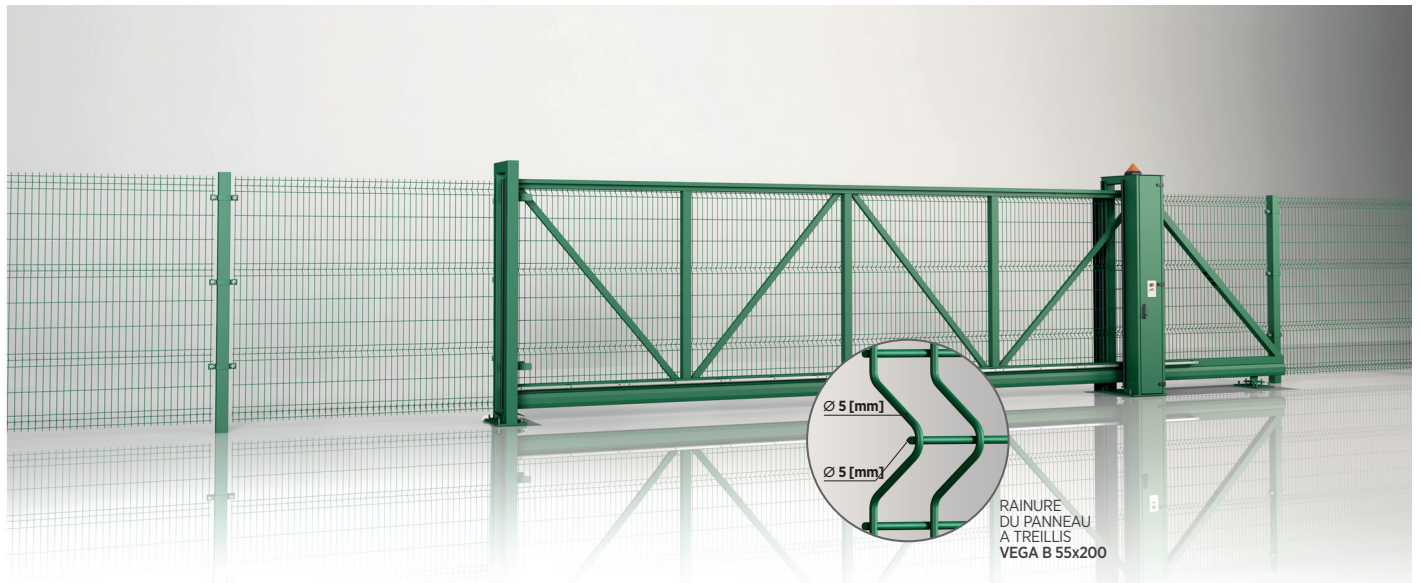
Clôture systémique avec portail coulissant PI 130 avec remplissage en panneaux à treillis VEGA B, maille 55x200
