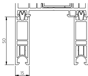
Podparapetní lišta 50 [mm]
