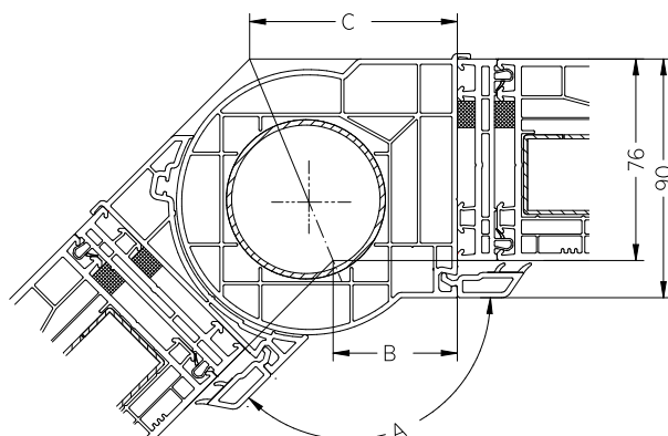
Trubková spojka 116.216 + rozšíření 15 mm
