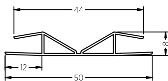
Profil spojení 50 [mm]
