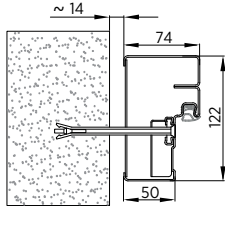
Obr. 68. Vložená zárubeň s přerušným tepelným mostem
