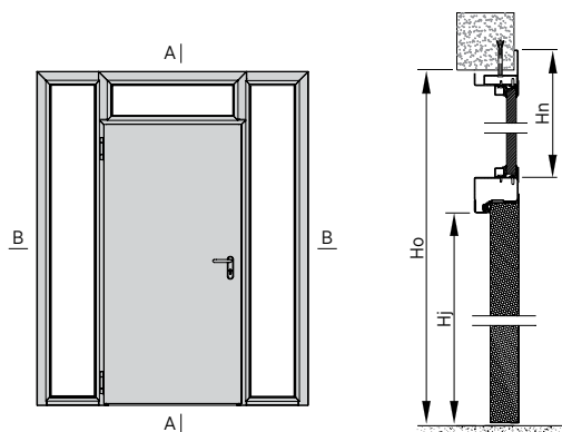
Obr. 101. Jednokřídlé dveře ECO s bočními světlíky a nadsvětlíkem
