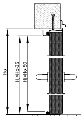
Obr. 109. Montáž jednokřídlých dveří s rohovou zárubní bez přerušného tepelného mostu do zdi – svislý řez
