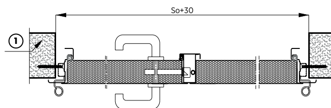
Obr. 112. Montáž dvoukřídlých dveří s rohovou zárubní bez přerušného tepelného mostu do ocelové konstrukce – vodorovný řez
