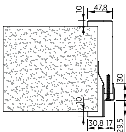
Obr. 136. Vložená zárubeň
