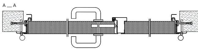
Obr. 64. Vodorovný řez na úrovni zámku exteriérovými plášťovými ocelovými dveřmi ECO s rohovou zárubní bez přerušeného tepelného mostu
