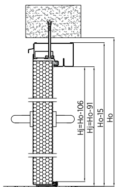
Obr. 126. Montáž dvoukřídlových dveří do zdi - vložena zárubeň s přerušeným tepelným mostem - svislý řez
