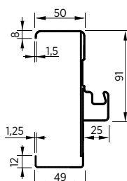
Obr. 159. Obložková zárubeň
