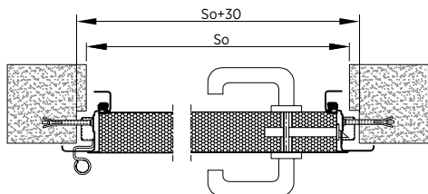
Obr. 107. Montáž jednokřídlých dveří s rohovou zárubní bez přerušného tepelného mostu do zdi – vodorovný řez
