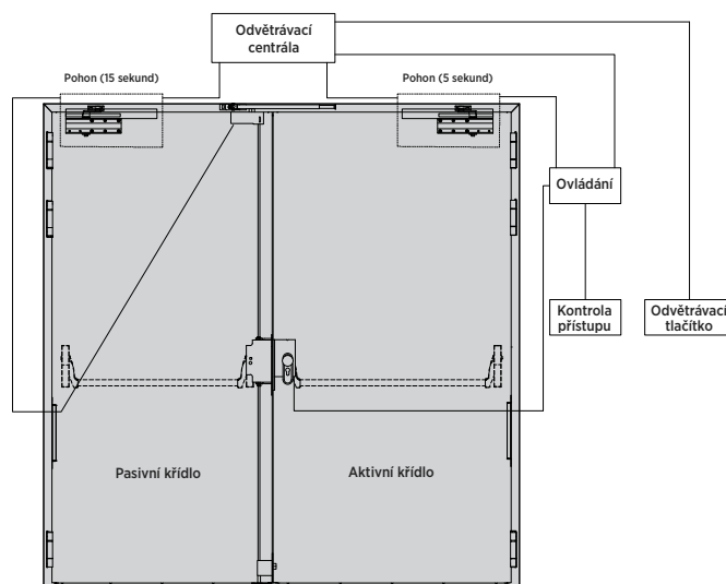
Obr. 100. Schéma zapojení prvků systému odvětrání dvoukřídlových plášťových ocelových dveří s panikovou funkcí
