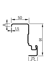
Obr. 157. Rohová zárubeň – standard
