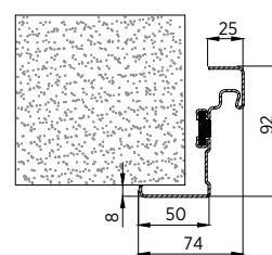
Obr. 31. Rohová zárubeň s přerušeným tepelným mostem.
