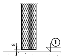
Obr. 71. Spodní mezera dveří bez prahu
