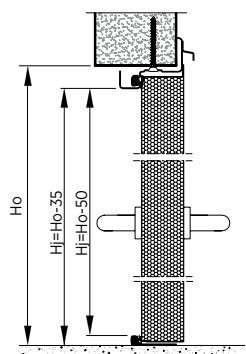
Obr. 113. Montáž jednokřídlých dveří s rohovou zárubní bez přerušného tepelného mostu do ocelové konstrukce – svislý řez
