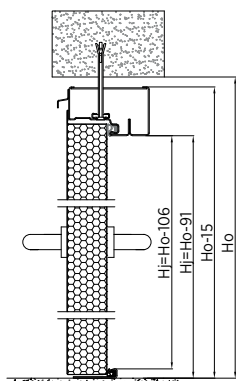
Obr. 124. Montáž jednokřídlových dveří do zdi - vložena zárubeň s přerušeným tepelným mostem - svislý řez
