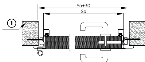
Obr. 111. Montáž jednokřídlých dveří s rohovou zárubní bez přerušného tepelného mostu do ocelové konstrukce – vodorovný řez
