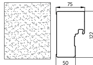
Obr. 29. Vložená zárubeň
