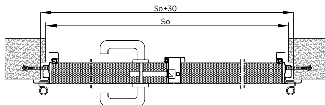
Obr. 108. Montáž dvoukřídlých dveří s rohovou zárubní bez přerušného tepelného mostu do zdi – vodorovný řez
