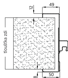
Obr. 30. Obložková zárubeň
