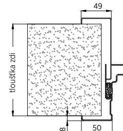
Obr. 33. Obložková zárubeň s přerušeným tepelným mostem
