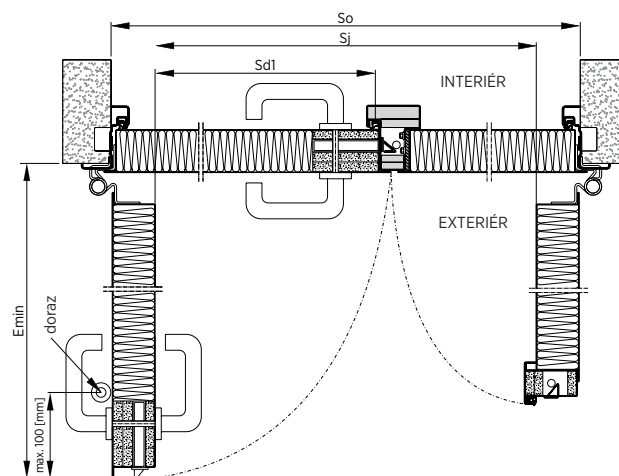
Obr. 177. Montáž dvoukřídlých dveří s rohovou zárubní – vodorovný řez
