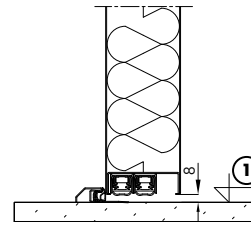
Obr. 35. Řešení s prahem a automatickým padacím prahem
