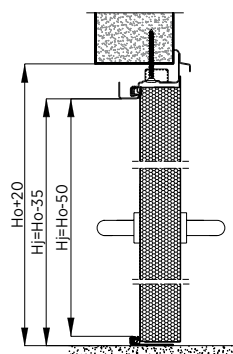
Obr. 114. Montáž dvoukřídlých dveří s rohovou zárubní bez přerušného tepelného mostu do ocelové konstrukce – svislý řez
