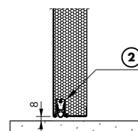
Obr. 72. Řez padacím prahem
