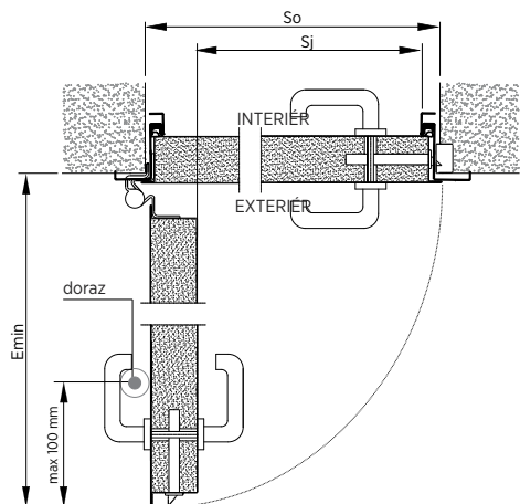
Obr. 127. Montáž před stavebním otvorem – rohová zárubeň bez přerušeného tepelného mostu – vodorovný řez
