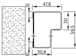
Obr. 135. Vložená zárubeň
