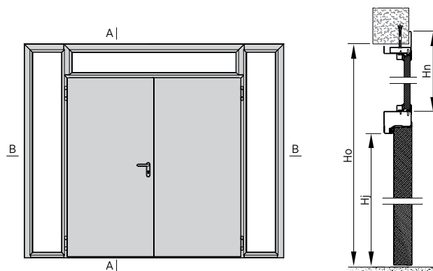
Obr. 104. Dvoukřídlé dveře ECO s bočními světlíky a nadsvětlíkem
