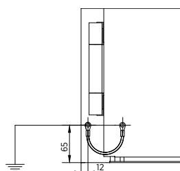
Obr. 96. Způsob provedení uzemnění dveří ECO
