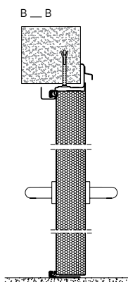
Obr. 60. Svislý řez exteriérovými plášťovými ocelovými dveřmi ECO s rohovou zárubní bez přerušeného tepelného mostu
