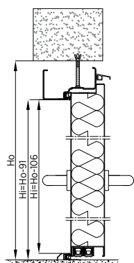
Obr. 45. Montáž jednokřídlých plášťových dveří ECO Tech s vloženou zárubní bez přerušného tepelného mostu do zdi – svislý řez
