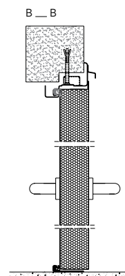
Obr. 63. Svislý řez dvoukřídlovými plášťovými ocelovými dveřmi ECO s rohovou zárubní bez přerušeného tepelného mostu
